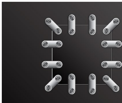
Ремонтна латка на наскрізний пробій
